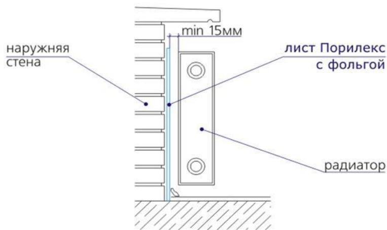
Рис. 2.1. Способ установки теплоотражающего экрана
